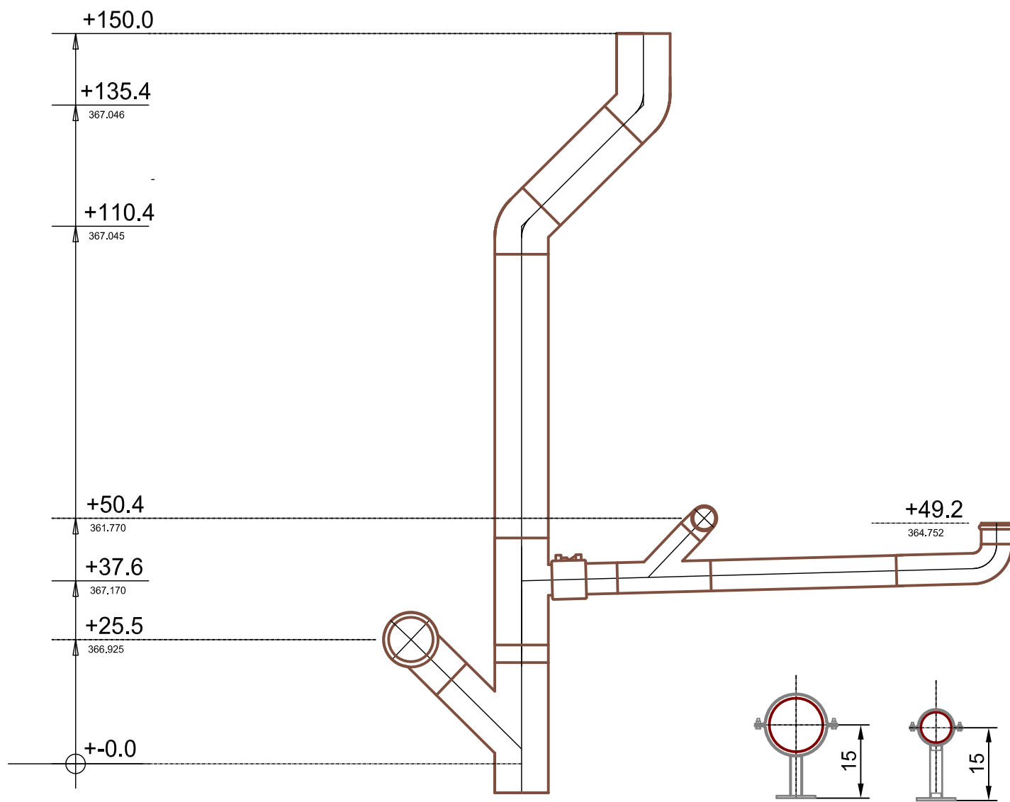
3 Rohrschellen \varnothing 110 und 1 Rohrschelle \varnothing 63
